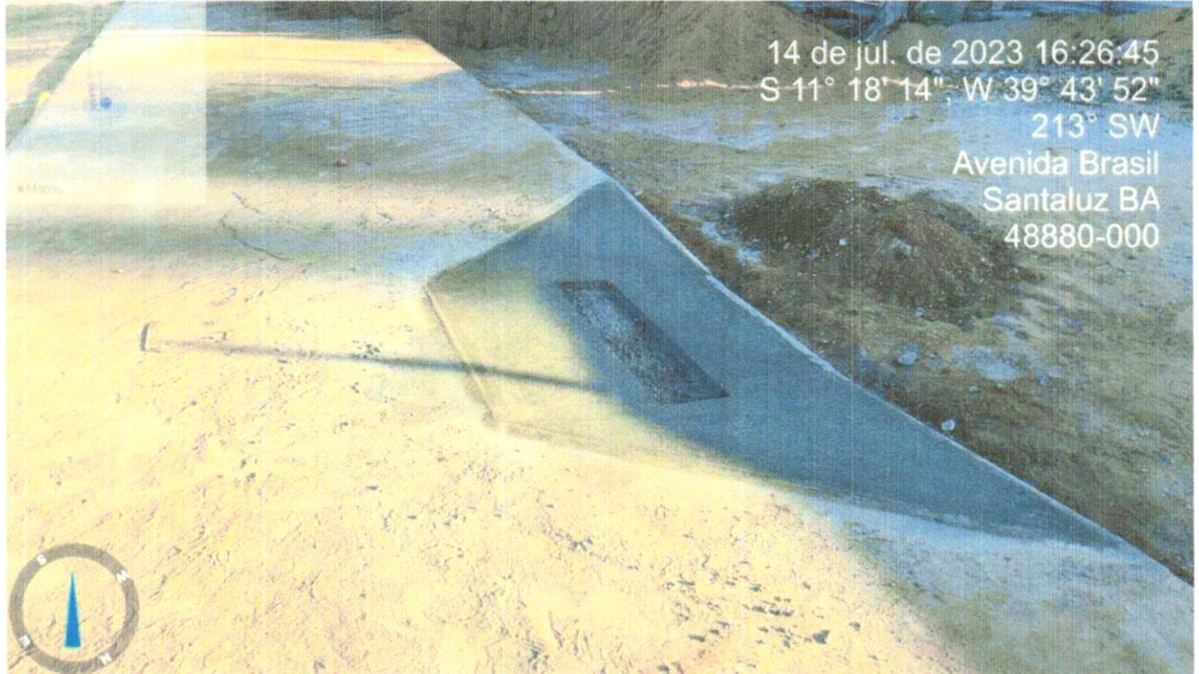
FOTO 12 - Rampa padrão para acesso de deficientes a passeio público, em concreto simples Fck=25MPa
